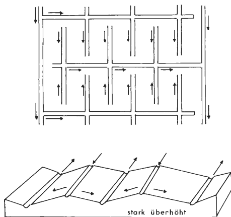
Abb. 17: Vielfältig verästeltetes Be- und Entwässerungssystem zur Düngung von Flößwiesen (nach HOFMANN 1985, aus POTT 1988a)
